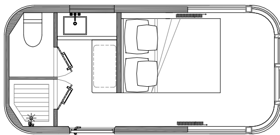
E3-II 平面布局图 — PLANE LAYOUT —
