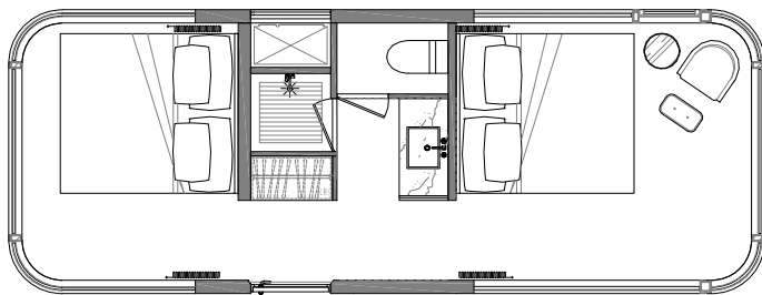
E6-II 平面布局图 — PLANE LAYOUT —
